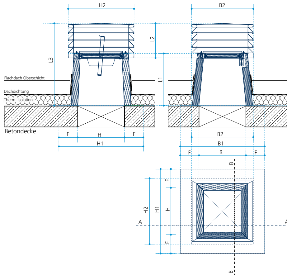
Schnitt B-B
