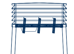
800 x 800 - 3 louvres
